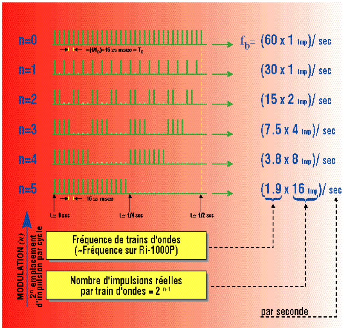
Fig. 6.1: Illustration des trains d'impulsions pour différentes valeurs de n , avec une fréquence de base, f_b , égale à 60 impulsions par seconde.
