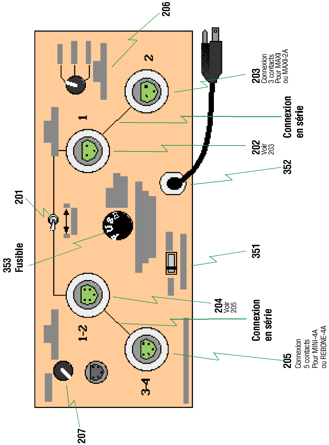
Fig. 4.4 Le Contrôleur RESC™, MBI-3000 (Panneau arrière)
